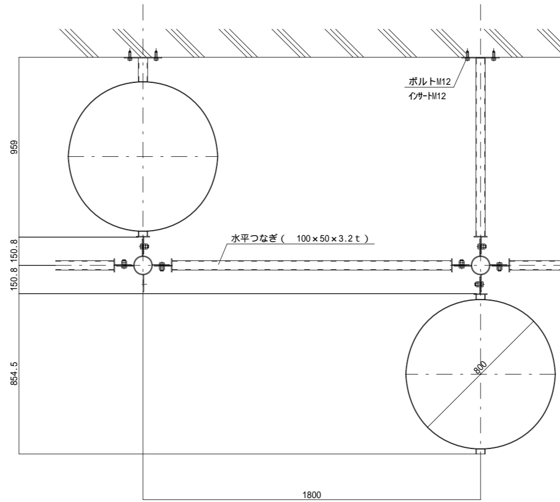
平面詳細図 S=1/20
